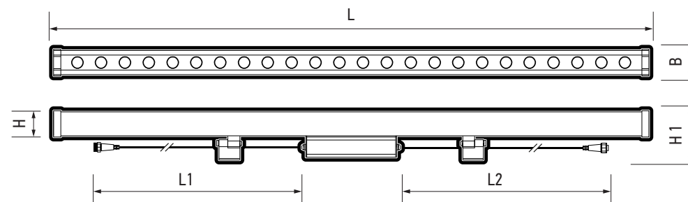
Рис.1 Светильник PWW
