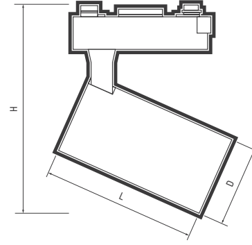
Рис.1 Проектор PTR 13
