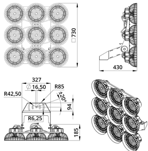
Габаритный чертёж
