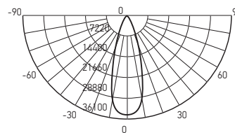
PTR 0620 20w
