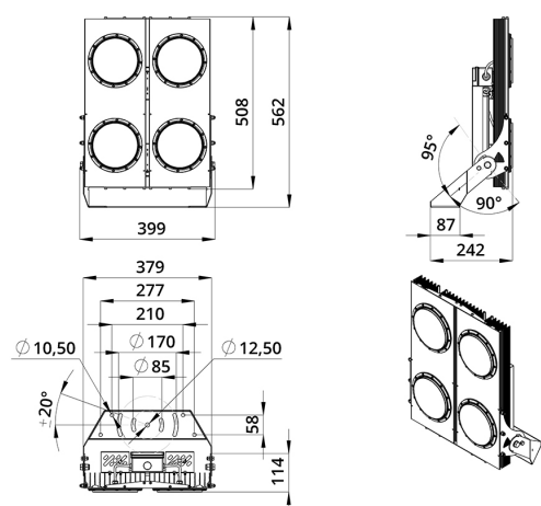
Габаритный чертеж
