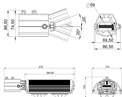
Габаритный чертёж
