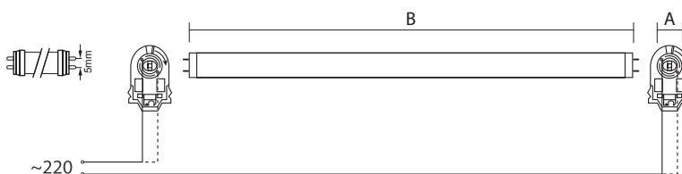
Схема подключения лампы PLED T5
