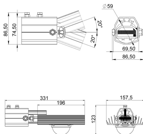
Габаритный чертеж
