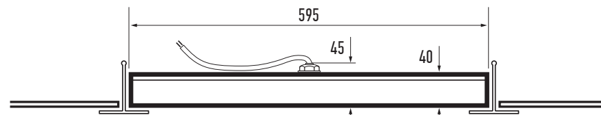
Рис.1 Светильник PPL SPEC1
