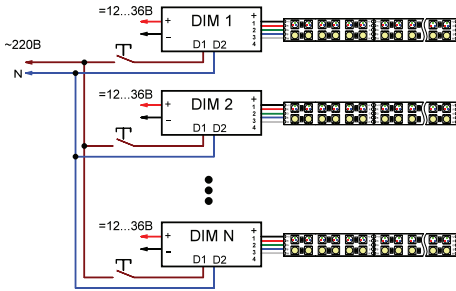
Рис.2. Использование управления DALI
